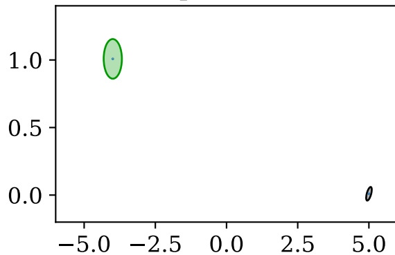
pmc fit
